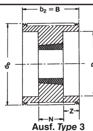
Ausf. Type 3
