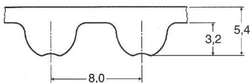
Typ 8M HP (tylko wartości średnie – mm)
