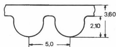
Typ 5M (tylko wartości średnie – mm)
