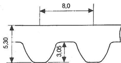
Typ S8M (tylko wartości średnie – mm)
