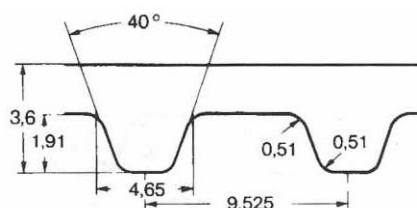
Type L (tylko wartości średnie – mm)
