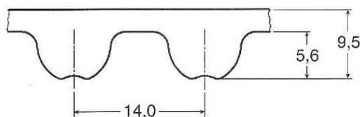
Typ 14M HP (tylko wartości średnie – mm)
