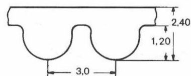
Typ 3M (tylko wartości średnie – mm)
