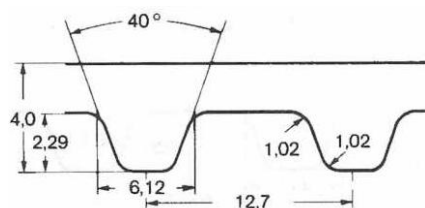
Type H (tylko wartości średnie – mm)
