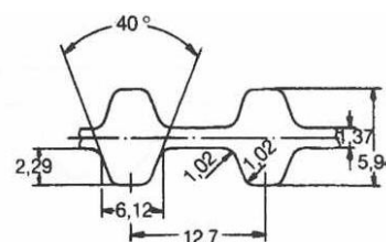
Typ DH (tylko wartości średnie – mm)
